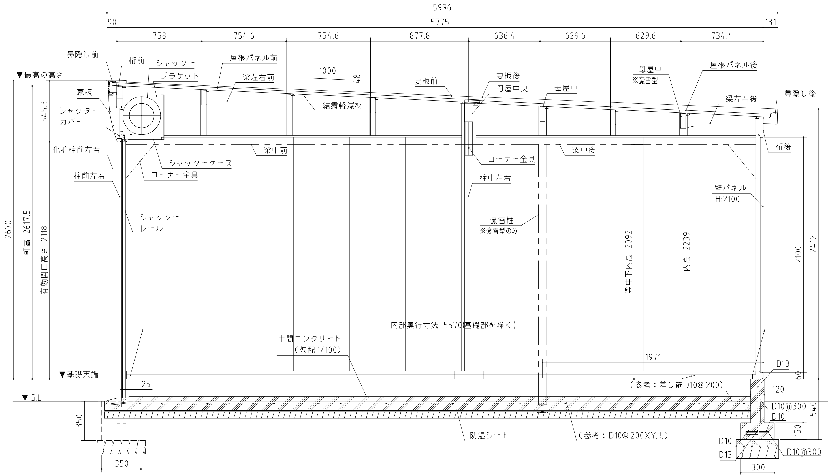
断面図(側面) <縮尺> S=1/20 ~一般型・豪雪型~ 機種名 DR-3157・3657HPA・HYA 3157・3657HPA・HYA-N[連棟数]
